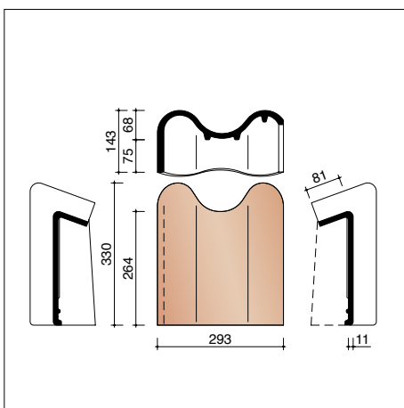
JOVH7580 Lanker gevelhaakvorst
