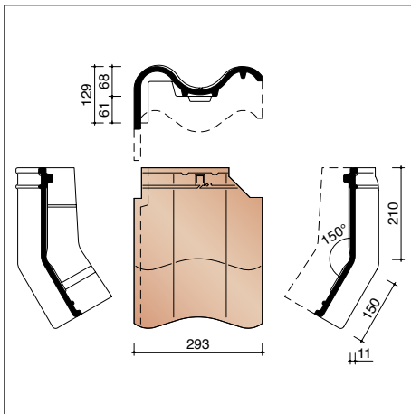
JOVH7280 Lanker gevelknikpan
