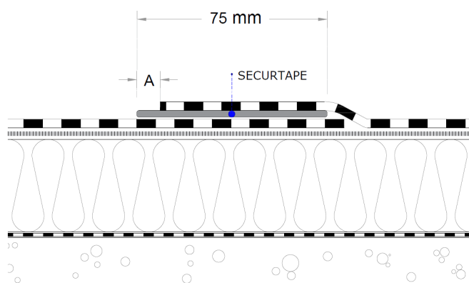
Fig. 4 – Joints réalisés au moyen de SECURTAPE™
