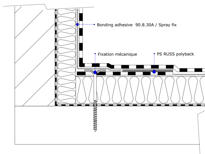
Fig. 3 – Exemple d'acrotère avec fixation au droit de l'angle
