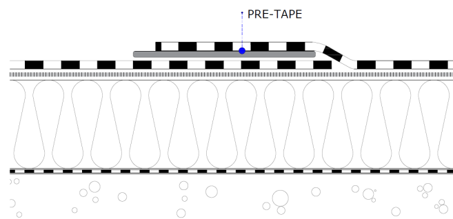
Fig. 5 – Joints réalisés au moyen de PRE-TAPE
