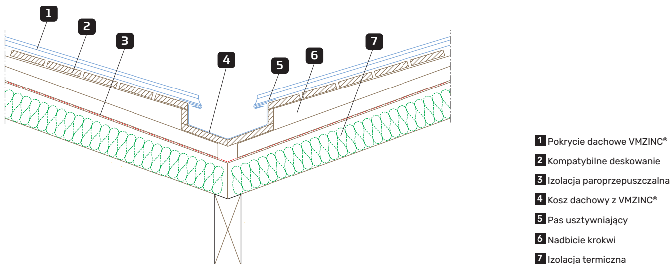
Rysunek 14b: Kosz wpuszczany
