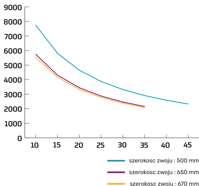
Wykres 1: Parametry systemu na rąbek stojący (VMZINC 0.7 mm; współczynnik bezpieczeństwa: 2,6)
