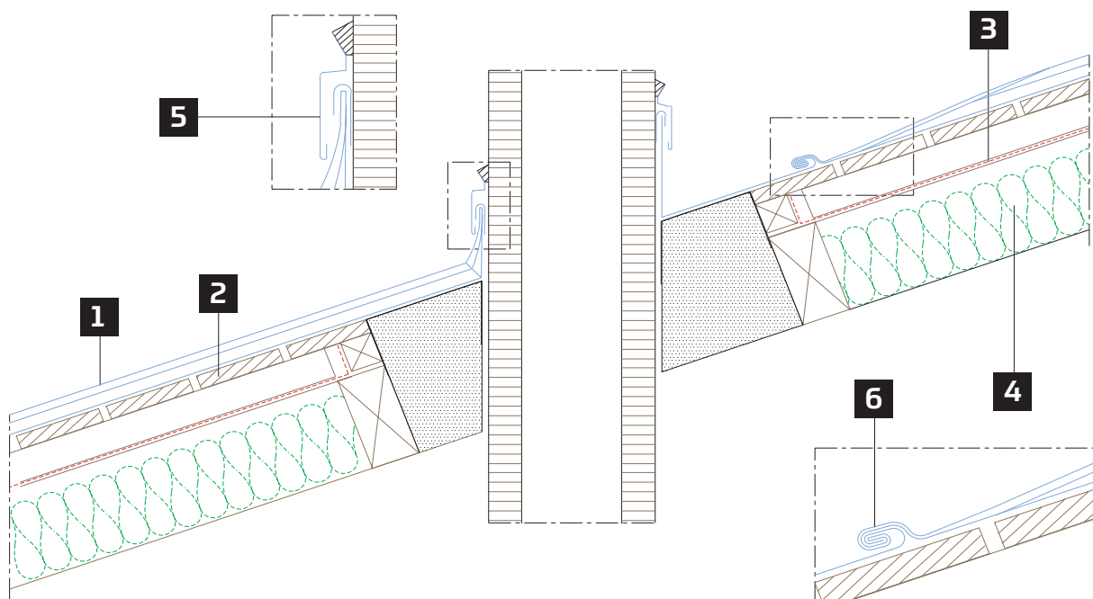
Rysunek 16a: Komin-przekrój poprzeczny
