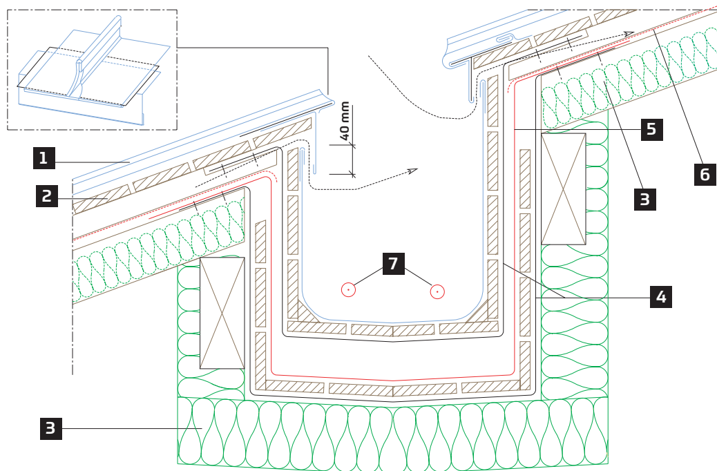
Rysunek 15: Koryto wpuszczane
