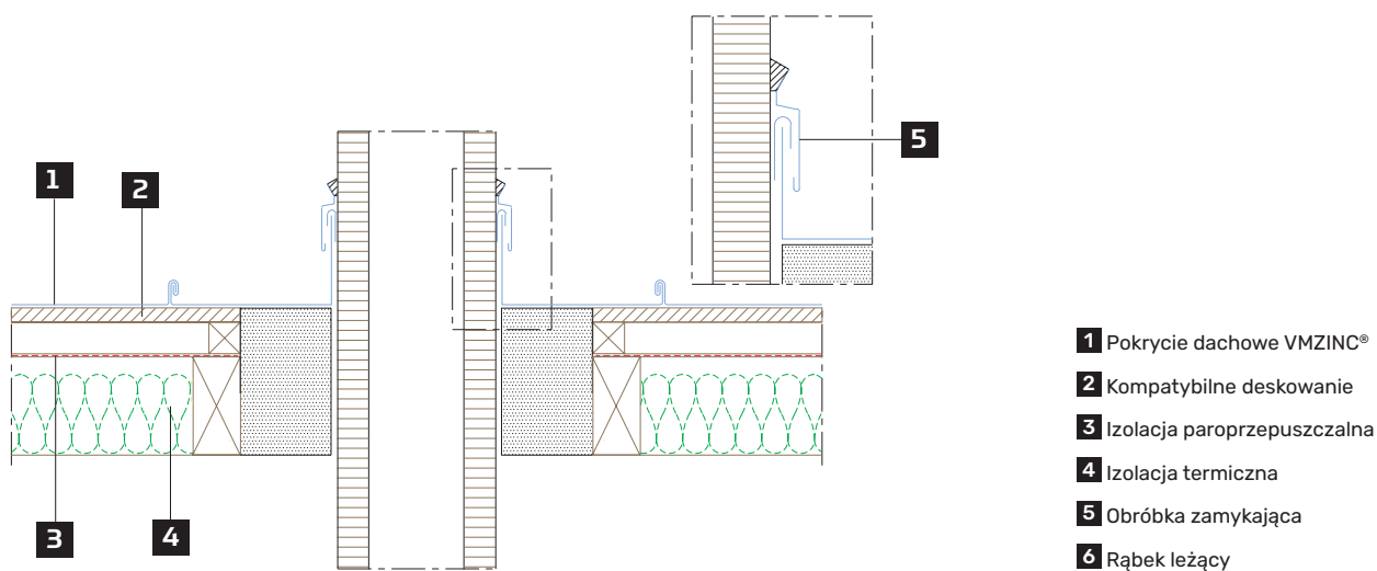
Rysunek 16b: Komin-przekrój podłużny
