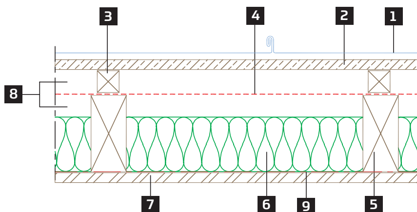
Rysunek 7. Tradycyjny system na rąbek stojący
