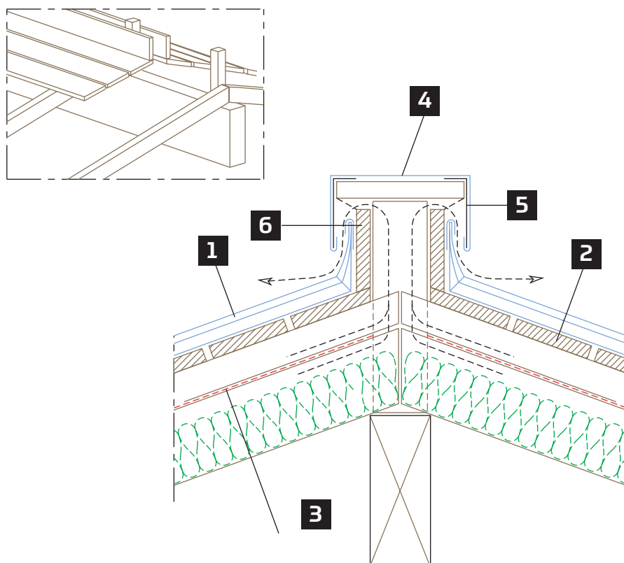
Rysunek 12: Kalenica
