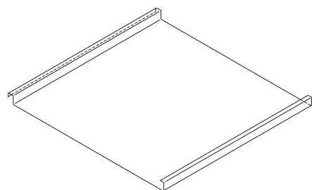
Rysunek 1 : Wyprofilowany arkusz na rąbek stojący
