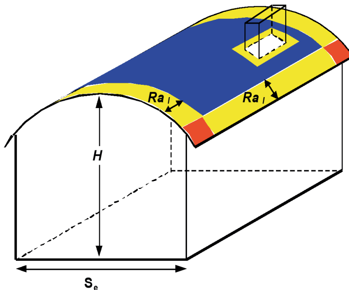
Rysunek 4: Powierzchnie narażone na większe obciążenia powodowane wiatrem
