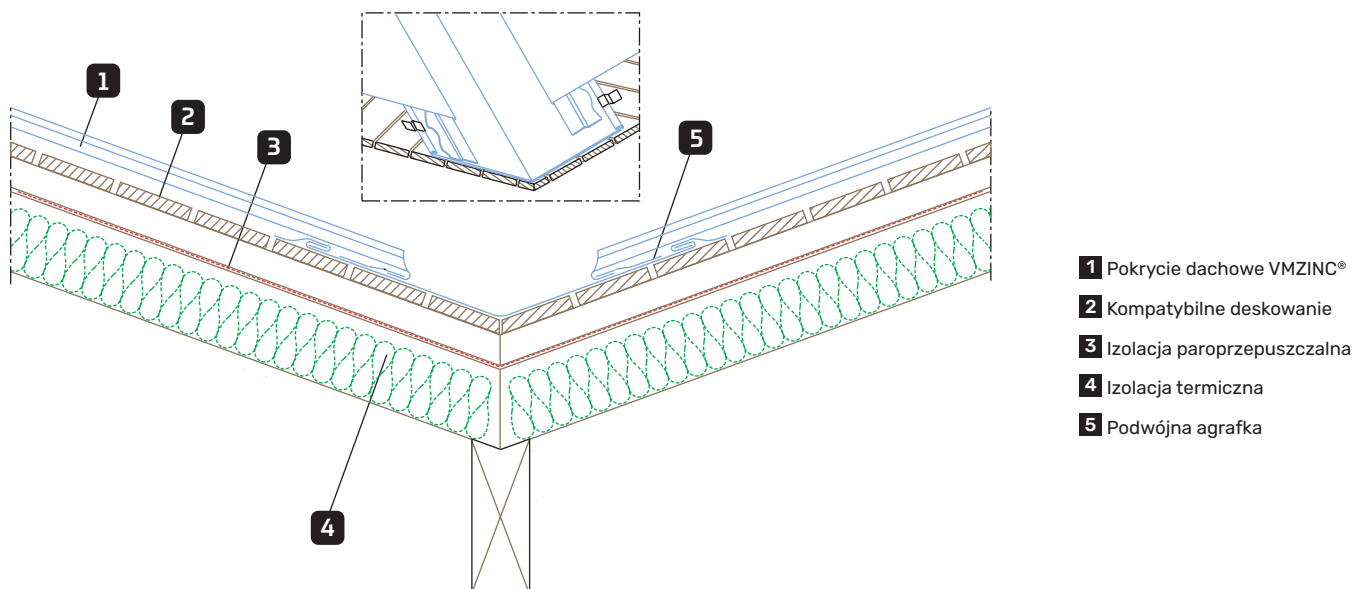
Rysunek 14a: Kosz z zabezpieczeniem
