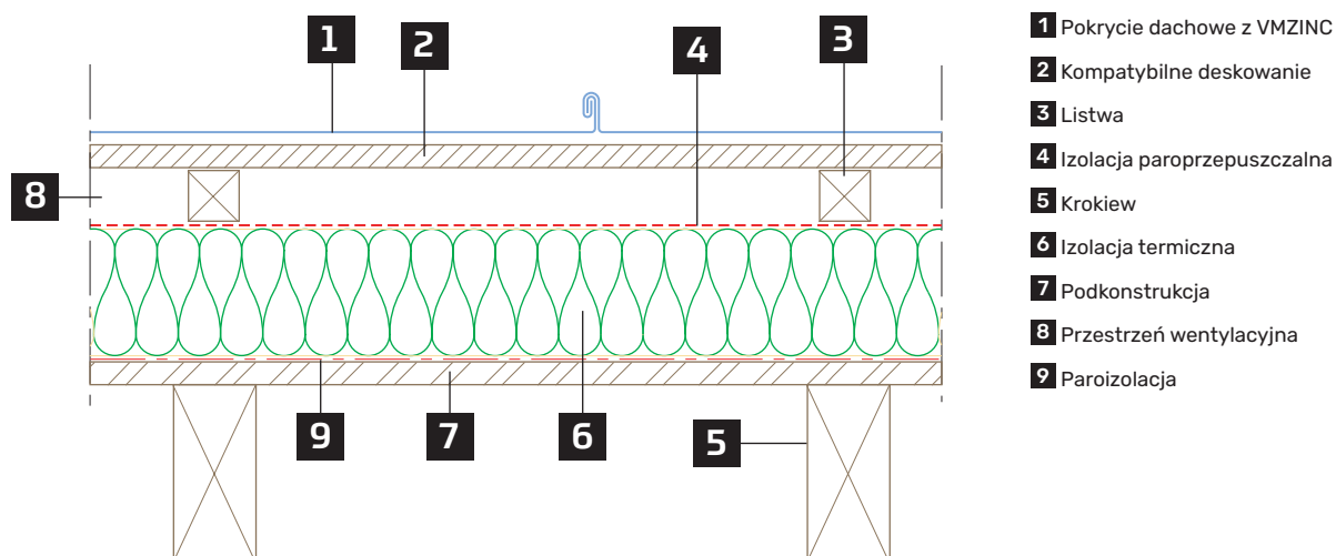
Rysunek 8: system SARKING
