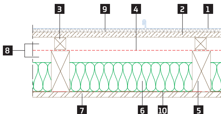
Rysunek 9: System DELTA VMZINC®
