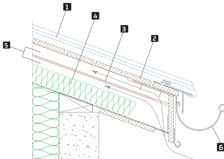
Rysunek 10: Okap
