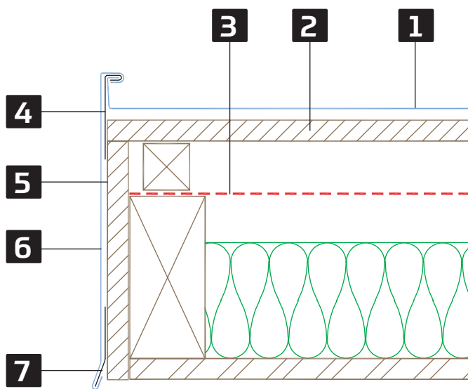
Rysunek 11: Krawędź szczytowa
