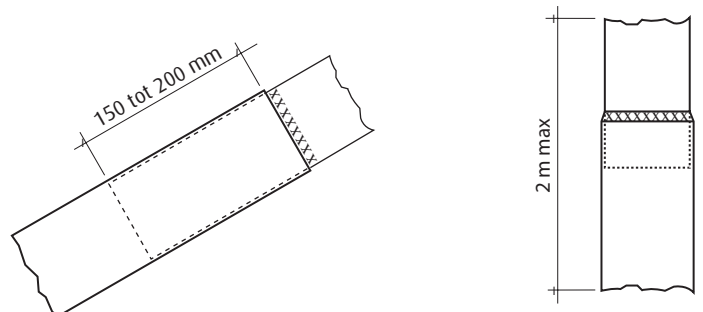
Recouvrement de 2 tuyaux obliques
