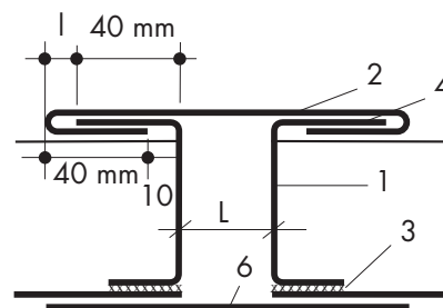
COUPE A-A
