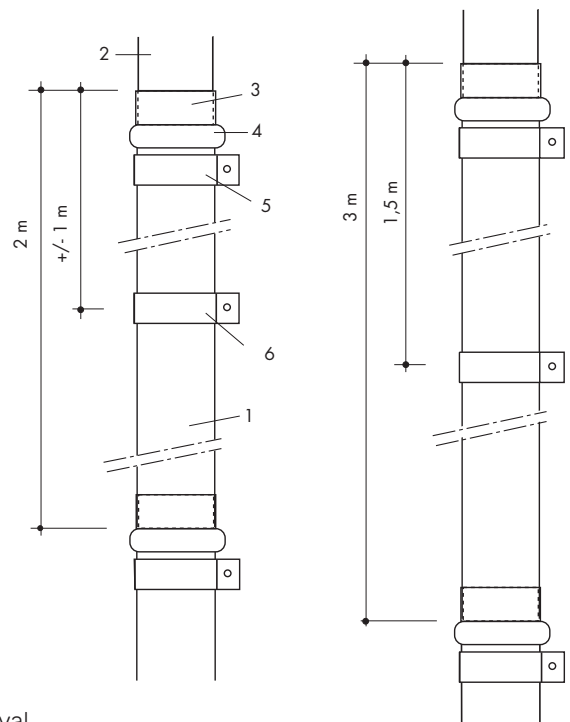
Bague autobloquante
