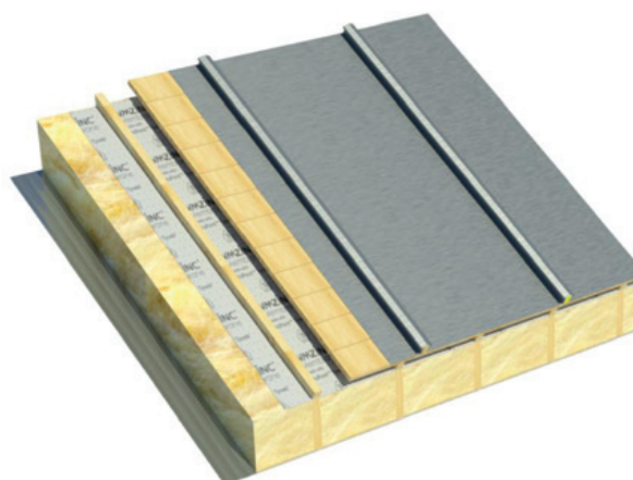
Tasseaux brevetés VMZINC sur support aéré
