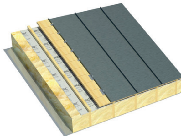
Joint debout VMZINC sur support aéré
