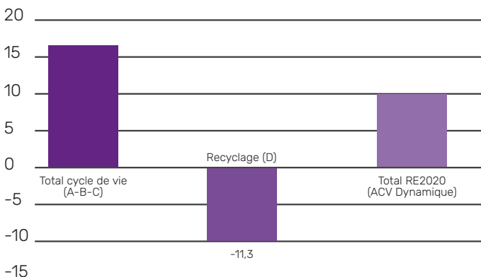
Impact sur le réchauffement climatique pour 1 m 2 de zinc laminé naturel VMZINC® en couverture Joint debout – Extrait de la FDES
