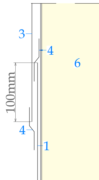
Coupe AA
